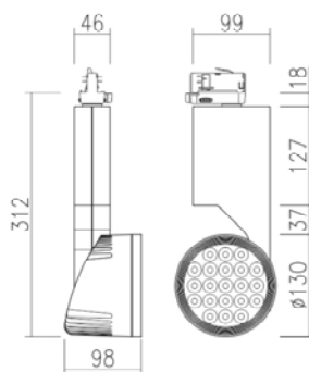
Technische Zeichnung
